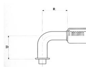
"O" ring-pijp zonder moer, 90° gebogen "O" ring tube connection, without nut, 90° elbow "O" ring tube connection, sans écrou, coudé 90°
