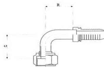
ORFS wartel - 90° elleboog ORFS female swivel - 90° elbow ORFS femelle tournant - coudé 90°
