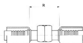
Verbindingsstuk met "Switch port" In line splicer with Switch port Splicer avec "Switch port"
