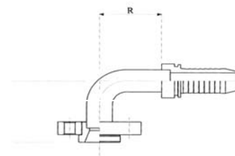
“Bock” flensaansluiting, 90° elleboog “Bock” flange connection, 90° elbow A bride “Bock” , coudé 90°
