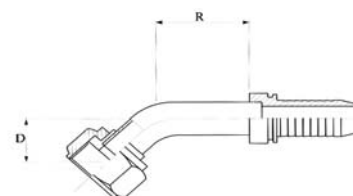
ORFS wartel - 45° elleboog ORFS female swivel - 45° elbow ORFS femelle tournant - coudé 45°
