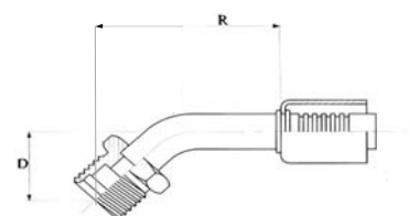
"O" ring buitendraad, 45° gebogen Male insert "O" ring, elbow 45° Raccord mâle "O" ring, coudé 45°
