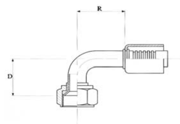
SAE 45° wartel - 90° elleboog SAE 45° flare swivel - 90° elbow Femelle tournant SAE 45° - coudé 90°
