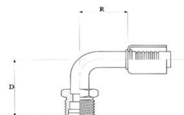
"O" ring buitendraad, 90° gebogen Male insert "O" ring, elbow 90° Raccord mâle "O" ring, coudé 90°
