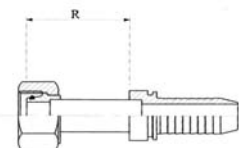
DIN 3865 - 24° Metrische wartel, lichte serie Metric swivel, light series Écrou tournant métrique, série légère
