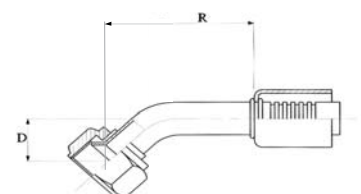
SAE 45° wartel - 45° elleboog SAE 45° flare swivel - 45° elbow Femelle tournant SAE 45° - coudé 45°
