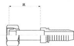
DIN 3863 - 60° Metrische wartel Metric swivel Écrou tournant métrique
