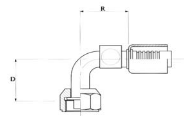
"O" ring wartel, met kijkglas, 90° gebogen "O" ring female swivel, with sight glass, elbow 90° "O" ring femelle tournant, avec "sight glass", coudé 90°
