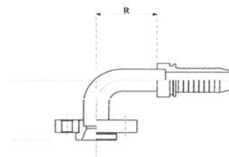
“Bock” flensaansluiting, 90° elleboog “Bock” flange connection, 90° elbow A bride “Bock” , coudé 90°
