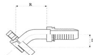
“Bock” flensaansluiting, 45° elleboog “Bock” flange connection, 45° elbow A bride “Bock” , coudé 45°
