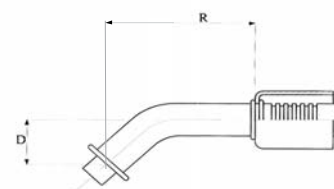
"O" ring wartel, 45° / R134 ventiel "O" ring swivel, 45°/ R134 valve "O" ring écrou tournant, 45° R134 valve
