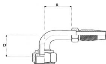
ORFS wartel - 90° elleboog ORFS female swivel - 90° elbow ORFS femelle tournant - coudé 90°
