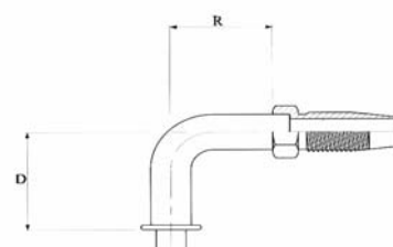
"O" ring-pijp zonder moer, 90° gebogen "O" ring tube connection without nut, 90° "O" ring tube connection sans écrou, 90°
