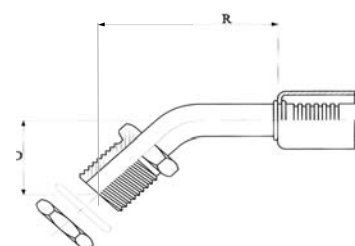
Schotdoorvoer "O" ring buitendraad, 45° gebogen Bulkhead male insert "O" ring, elbow 45° Raccord de cloison mâle "O" ring, coudé 45°
