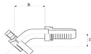
“Bock” flensaansluiting, 45° elleboog “Bock” flange connection, 45° elbow A bride “Bock” , coudé 45°
