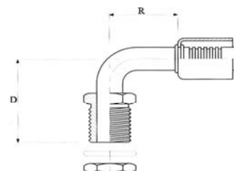
Schotdoorvoer "O" ring buitendraad, 90° gebogen Bulkhead male insert "O" ring, elbow 90° Raccord de cloison mâle "O" ring, coudé 90°
