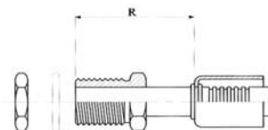
Schotdoorvoer "O" ring buitendraad, recht Bulkhead male insert "O" ring straight Raccord de cloison mâle "O" ring
