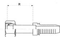
DIN 3865 - 24° Metrische wartel, lichte serie Metric swivel, light series Écrou tournant métrique, série légère
